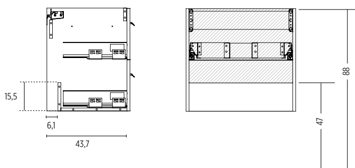
MEUBLES 2 TIROIRS
